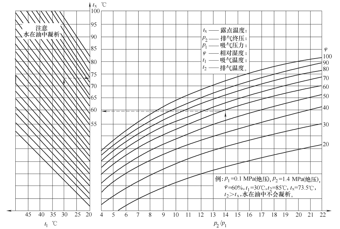
图 A.1 压缩空气露点温度
