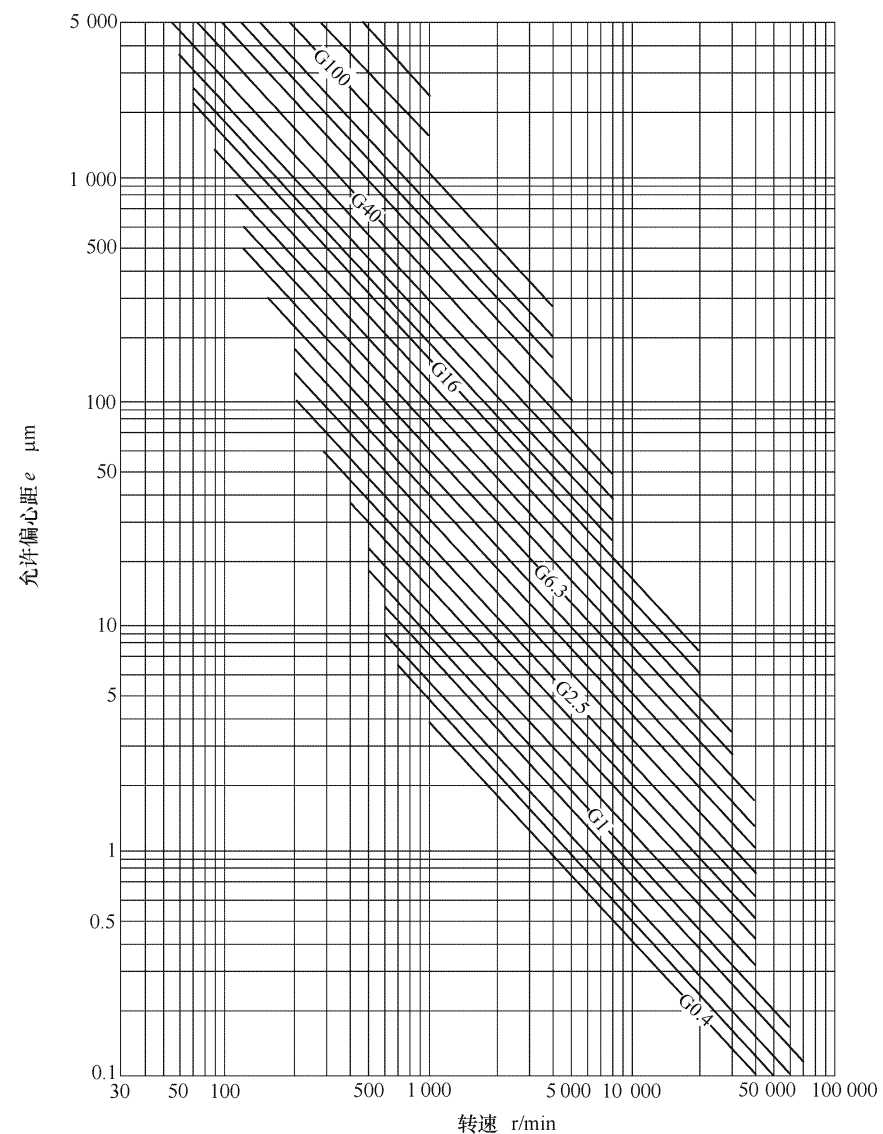
图 B.1 允许偏心距
